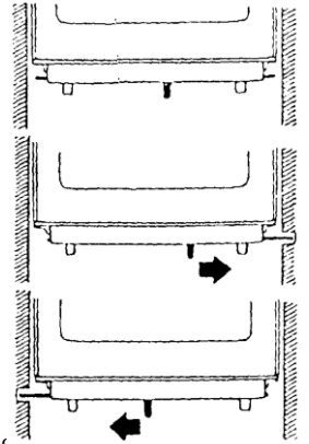
Esquemas: funcionamento da barra anti-oscilação
