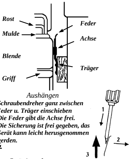
Abb. Stabilisatorriegel
