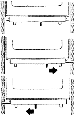
Schemor: krängningshämarens funktion
